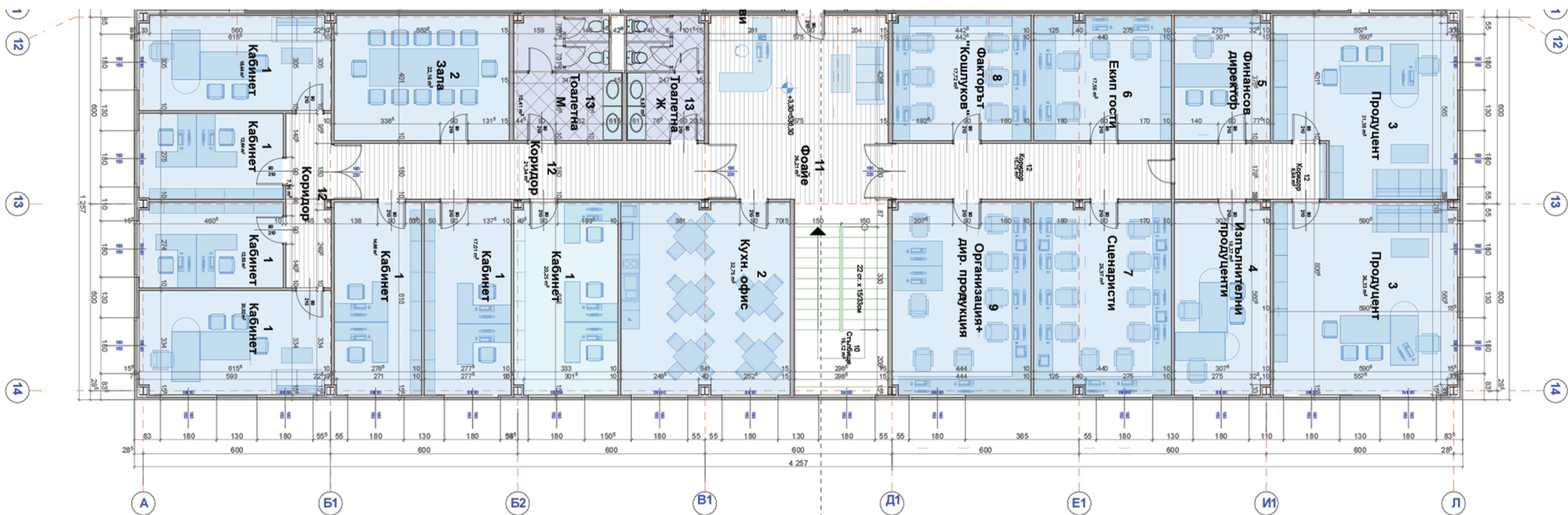
РАЗПРЕДЕЛЕНИЕ НА КОТА + 3.30
